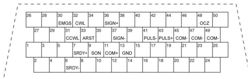
ASDA-A2 (50 Pins)
