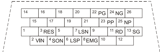
MR-E (26 Pins)
