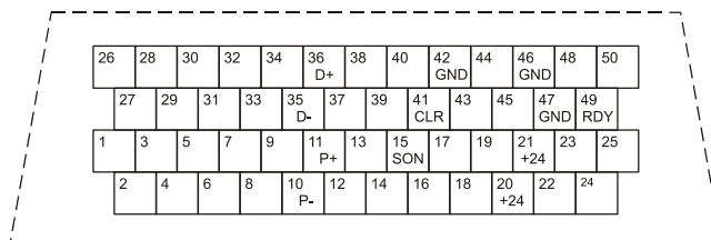
MR-JE (50 Pins)
