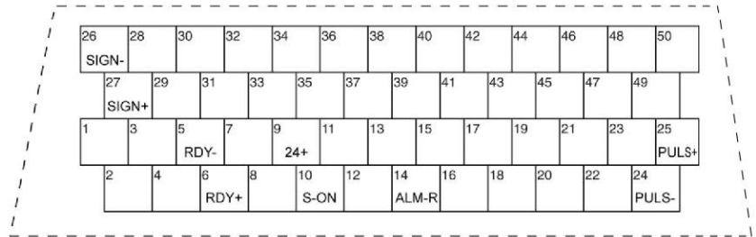
EDB (50 Pins)
