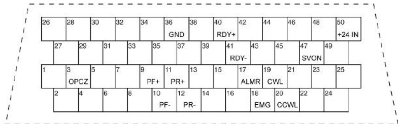
APD-VS (50 Pins)
