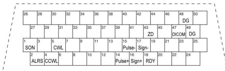
JSDA (50 Pins)
